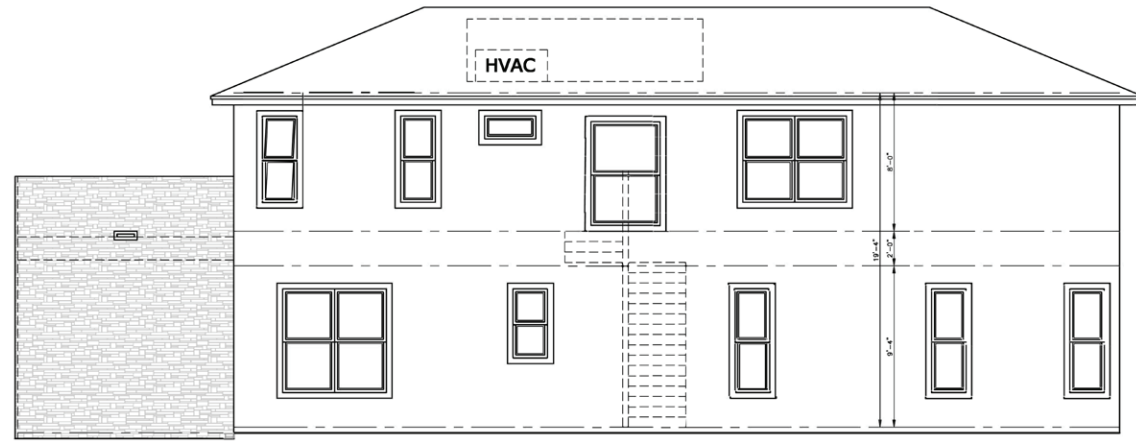
Right Elevation
