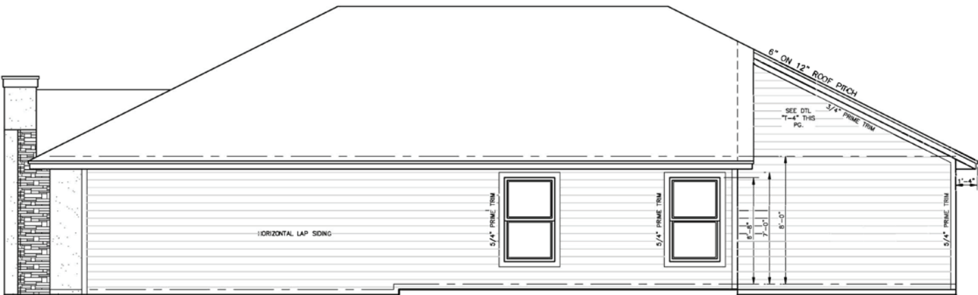
Right Elevation
